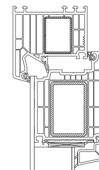
2 Profilschnitt Veka 82er Haustür als Aufsatzfüllung
