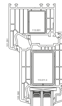
2 Profilschnitt Veka 82er Haustür als Einsatzfüllung
